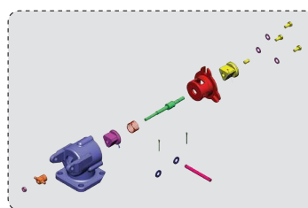
Блок выпускного клапана
