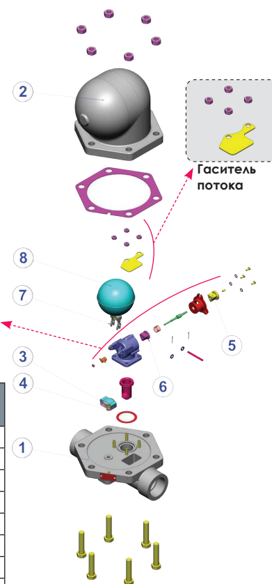
Блок выпускного клапана
